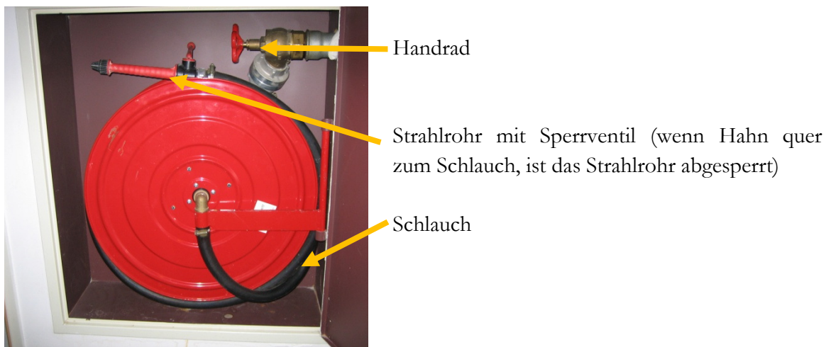
Abbildung 3: geöffneter Wandhydrantenkasten
