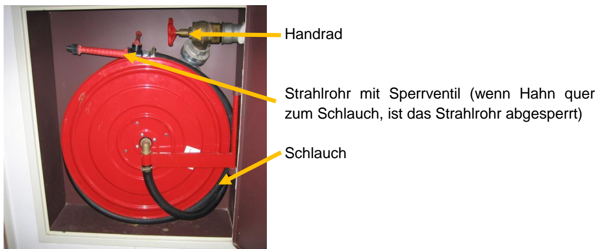
Abbildung 5: geöffneter Wandhydrantenkasten
