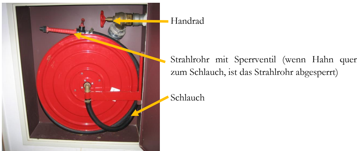
Abbildung 5: geöffneter Wandhydrantenkasten
